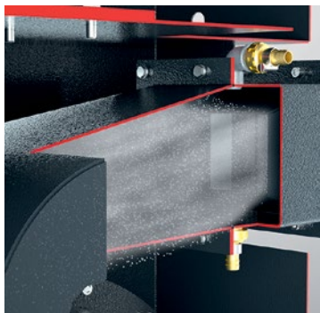
Schnittbild: In der Bedüsungzone entsteht ein dichter Wassertropfenschleier
