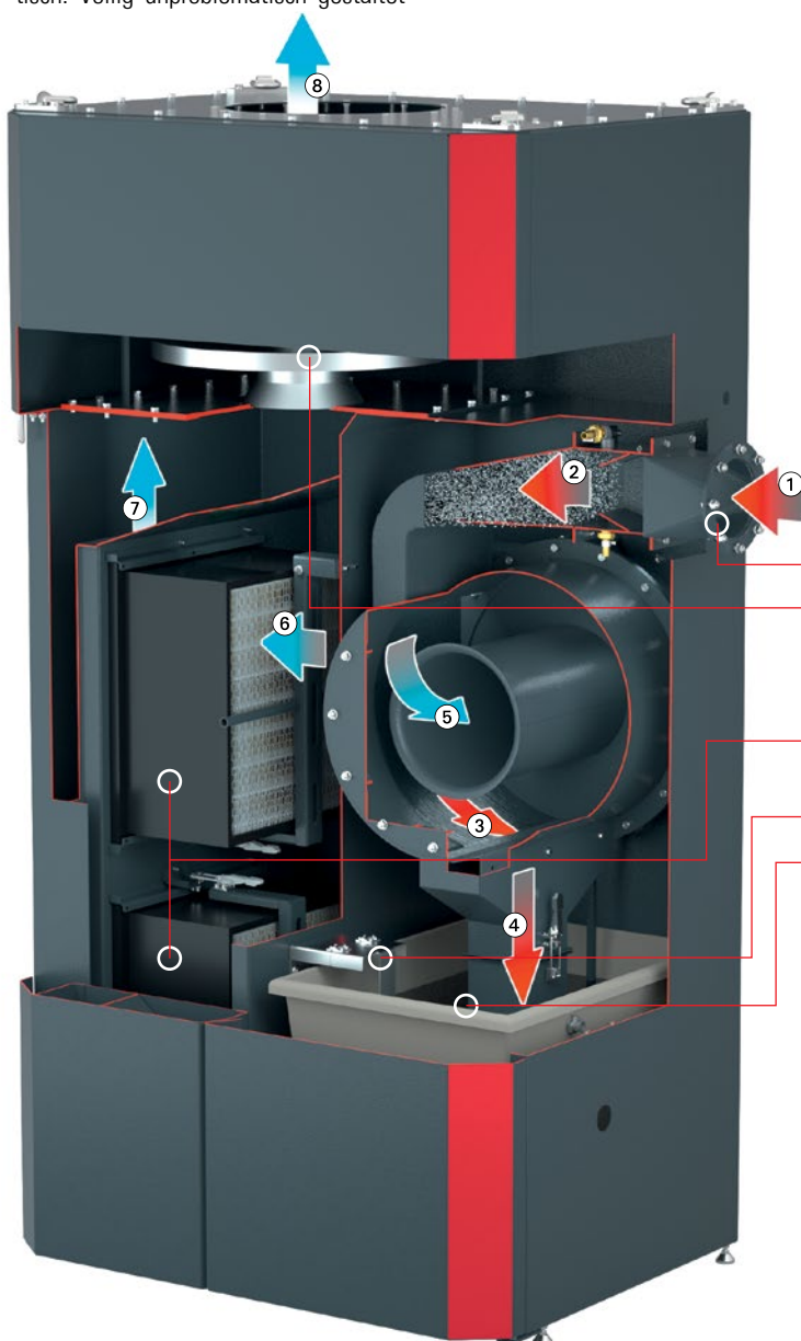
HydronPlus mit glattflächigem Gehäusedesign und geringem Platzbedarf (Breite 1250, Tiefe 946, Höhe 2430, in mm)
