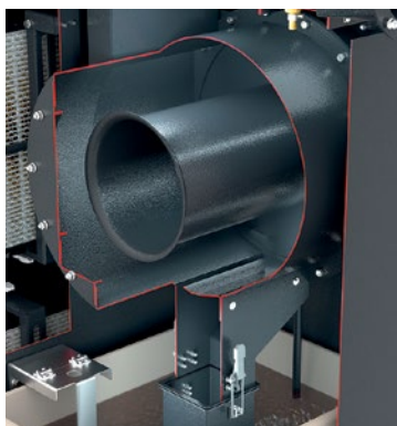
Schnittbild: Tropfenabscheider und Tauchrohr zur Abführung des Prozesswassers in den Prozesswasserbehälter
