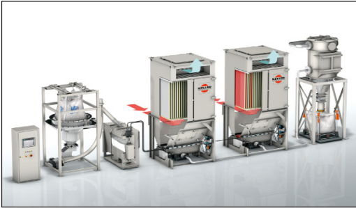
RECLAIM Filtertechnik mit zentraler BIG-BAG Ver- und Entsorgung
