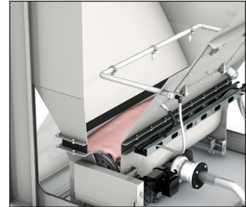
Fluidrotor: Höchste Funktionszuverlässigkeit durch mechanische Precoat-Fluidisierung
